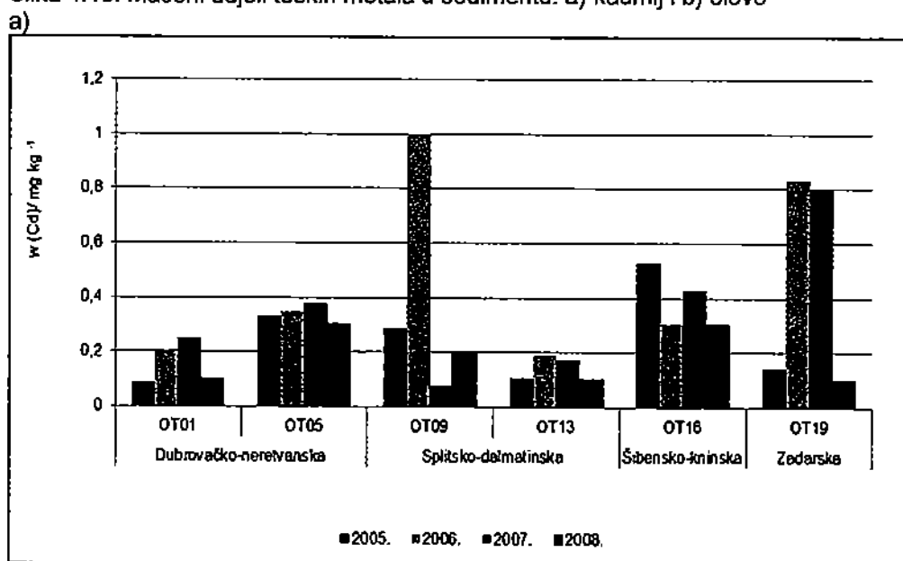
Slika 4.13. Maseni udjeli teških metala u sedimentu: a) kadmij i b) olovo
