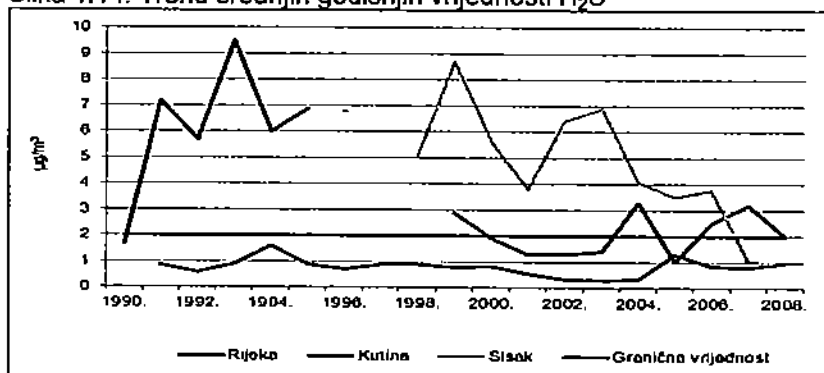
Slika 1.14. Trend srednjih godišnjih vrijednosti \text{H}_2\text{S}
