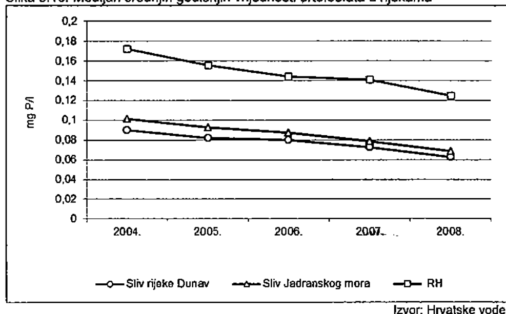
Slika 3.10. Medijan srednjih godišnjih vrijednosti ortofosfata u rijekama
