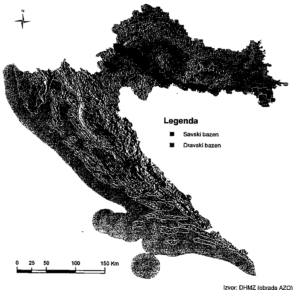
Slika 3.2. Karta piezometara na slivovima Save i Drave
