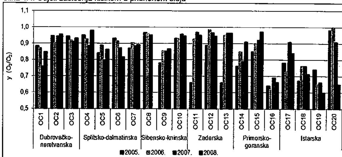
Slika 4.4. Udjeli zasićenja kisikom u pridnom sloju
