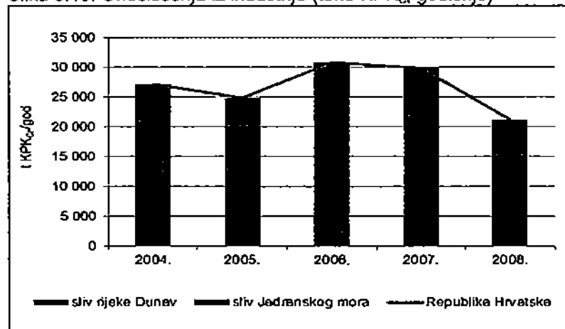
Slika 3.19. Onečišćenja iz industrije (tone KPK_{Cr} godišnje)
