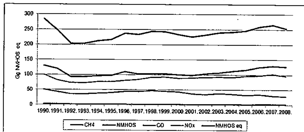
Slika 1.4. Trend emisije prethodnika ozona (Gg NMHOS eq) 117
