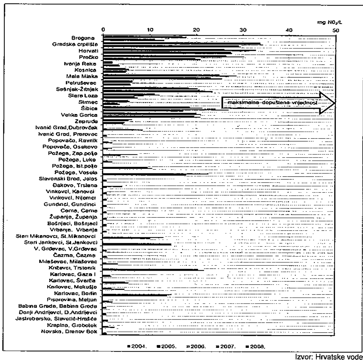
Slika 3.15. Medijan srednjih vrijednosti koncentracije nitrata na vodočrpilištima sliva Save
