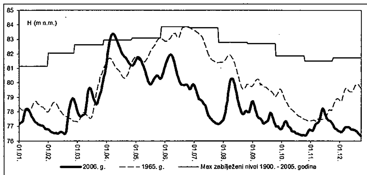
Slika 3.28. Rijeka Dunav, stanica Vukovar - nivogram 148 1965. i 2006. godine
