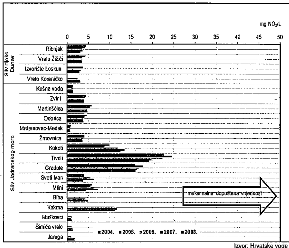
Slika 3.16. Srednje vrijednosti koncentracije nitrata na području krša (kaptirana izvorišta i bunari)
