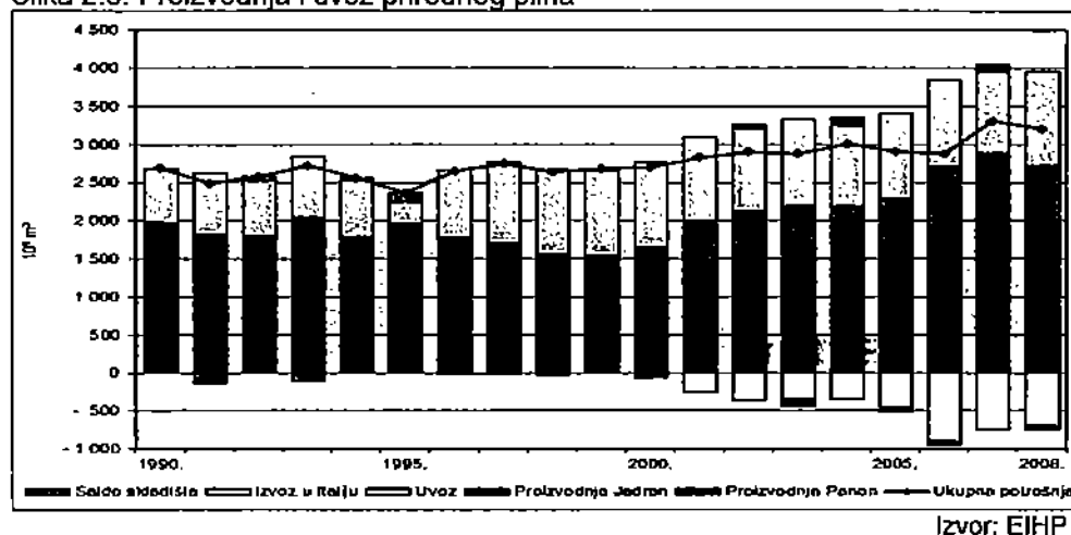
Slika 2.6. Proizvodnja i uvoz prirodnog plina
