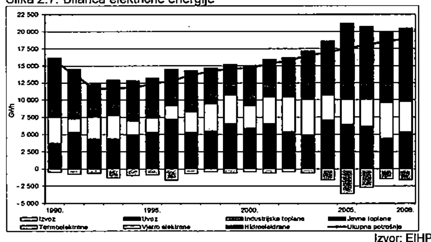
Slika 2.7. Bilanca električne energije
