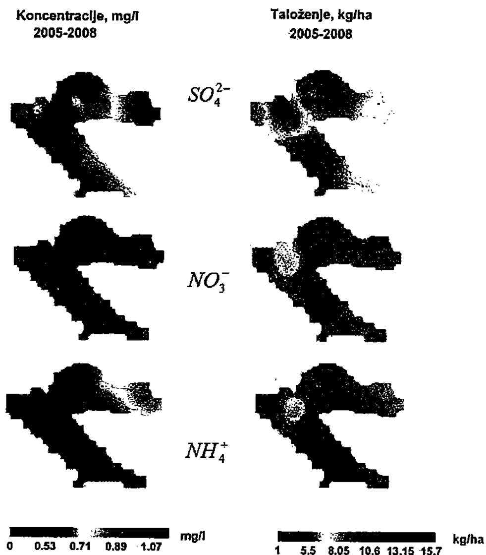
Slika 1.10. Prostorna razdioba srednjih godišnjih koncentracija (mg/l) i srednjega godišnjeg taloženja (kg/ha) iona sulfata ( \text{SO}_4^{2-} ), nitrata ( \text{NO}_3^- ) i amonija ( \text{NH}_4^+ ) za razdoblje od 2005. do 2008. Korištena je Kriging-interpolacijska metoda (Matheron, 1963.).
