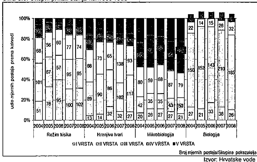
Slika 3.6. Ukupni prikaz stanja kakvoće vode
