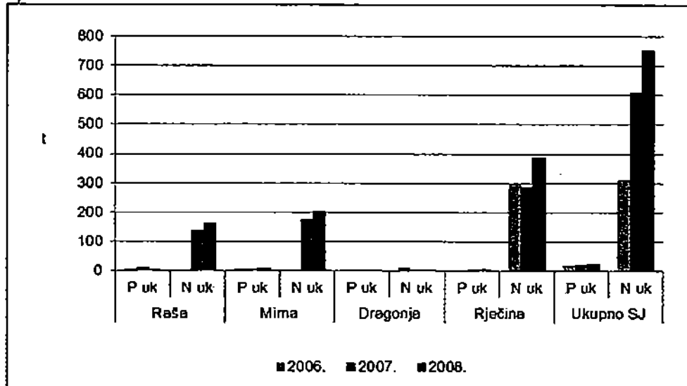
Slika 4.8. Godišnji unos hranjivih tvari glavnim vodotocima: a) sjeverni Jadran i b) južni Jadran
