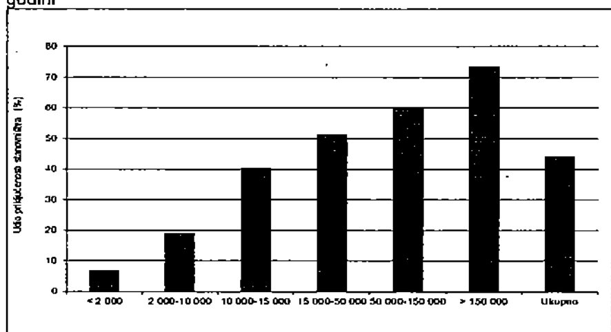
Slika 3.20. Priključenost stanovništva na sustav javne odvodnje prema veličini aglomeracije 143 u 2008. godini
