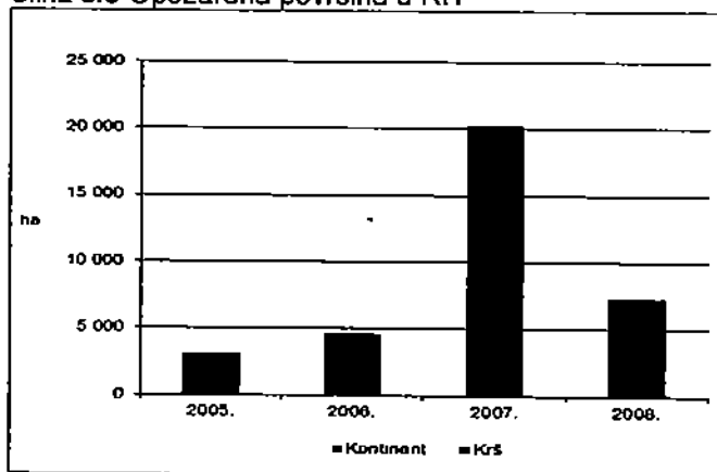
Slika 5.5 Opožarena površina u RH
