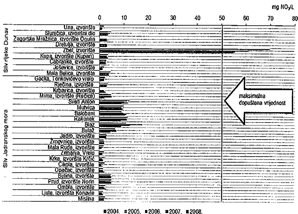
Slika 3.17. Srednje godišnje vrijednosti nitrata u izvoristima
