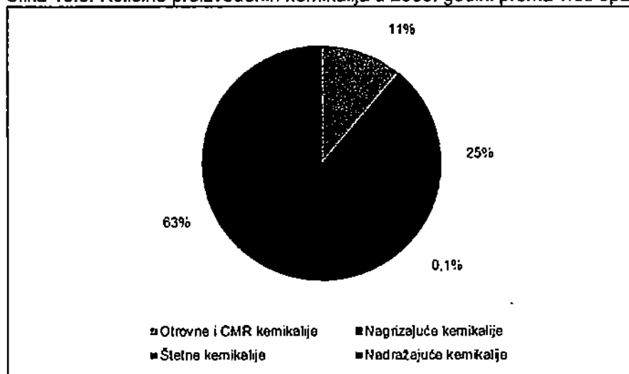
Slika 10.3. Količine proizvedenih kemikalija u 2008. godini prema vrsti opasnosti za ljudsko zdravlje
