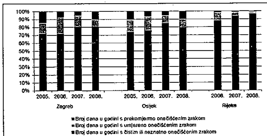
Slika 1.13. Kakvoća zraka u urbanim područjima: PM 10 (ukupno u %)
