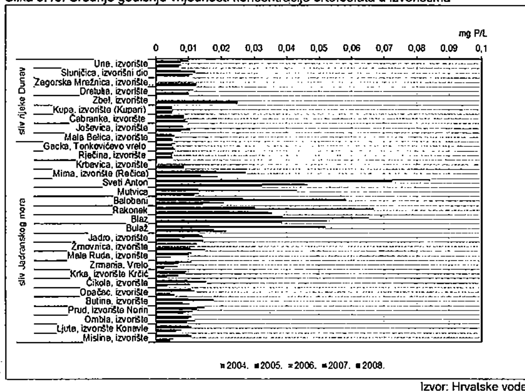
Slika 3.18. Srednje godišnje vrijednosti koncentracije ortofosfata u izvorima
